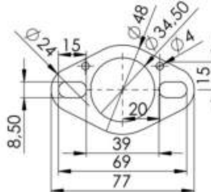
S.s. flange Cod.206443R
