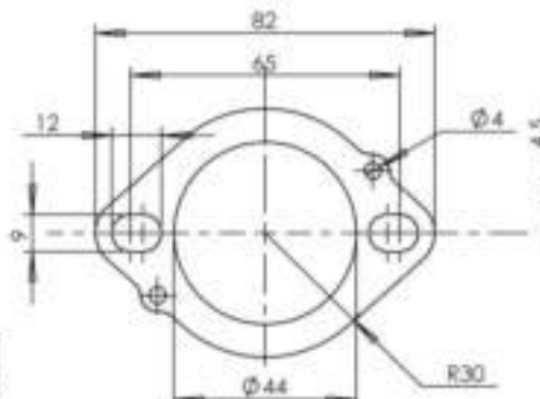
Flange kit Cod.204569R
