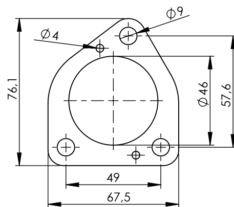
Flange s.s. sp.6mm cod.207016
